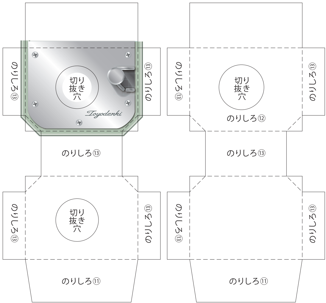
マスコンボックス上パーツ
