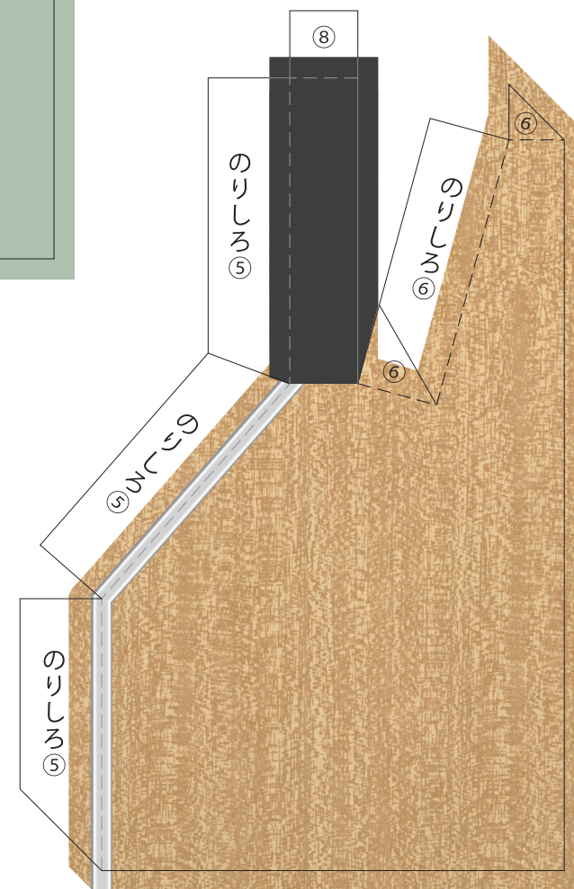
側面パーツ
