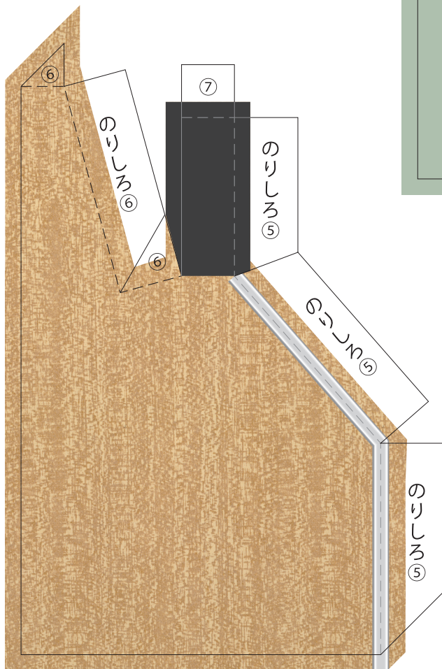
側面パーツ
