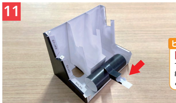
11 8で作ったマスコンパーツを台座側に入れる(向きに注意)
